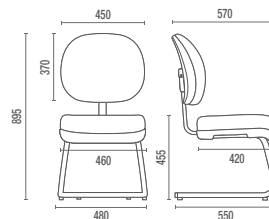
8207 S Executiva Aproximação
