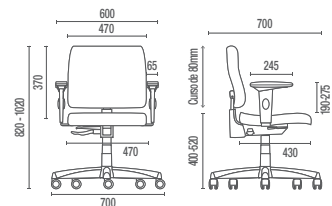
18004 SRE Executiva Giratória
