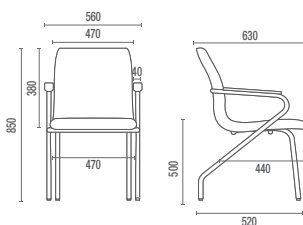
18006 Z Aproximação Fixa
