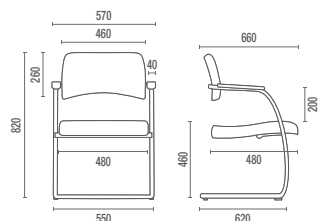
18007 S Secretária Aproximação
