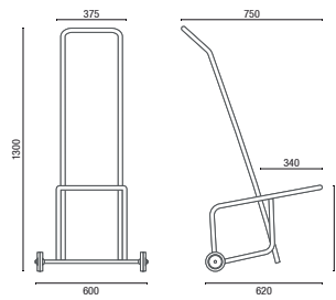
1100 Carrinho para Transporte
