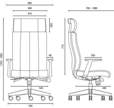
20.501 Presidente Giratória Braços fixos em Alumínio
